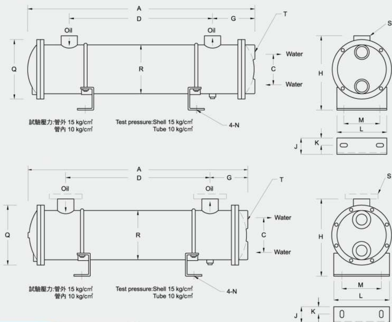
外型尺寸表
